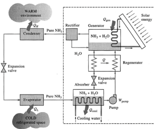
รูปที่ 1 วงจรการทำงานของเครื่องทำความเย็นชนิดดูดซึมโดยใช้สารละลายแอมโมเนียกับน้ำ [1]
