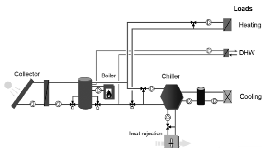
รูปที่ 3 ผังภูมิแสดงการติดตั้งระบบทำความร้อน ผลิตน้ำร้อน และ ทำความเย็น โดยใช้พลังงานแสงอาทิตย์ขนาดเล็กสำหรับครัวเรือน [10]
